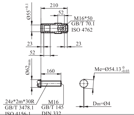
GFV/GFVZ/GFVF77输出轴
