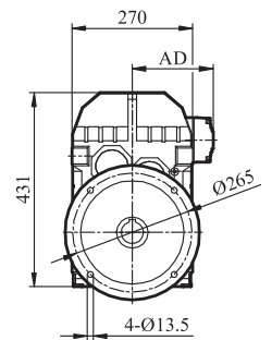
GFV/GFVZ/GFVF77输出轴
