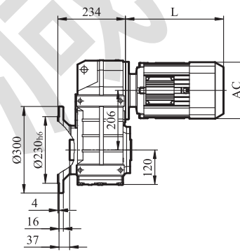
GFH/GFHZ/GFHF77输出轴
