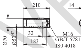
GFA/GFAZ/GFAF77输出轴
