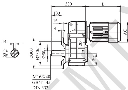
GFA/GFAZ/GFAF77输出轴
