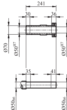
GFH/GFHZ/GFHF77输出轴
