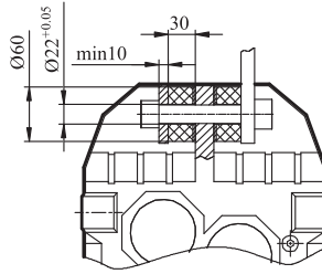
GFAZ/GFHZ/GFVZ77
